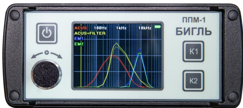
Рис.16 Экран тестовой проверки исправности каналов
