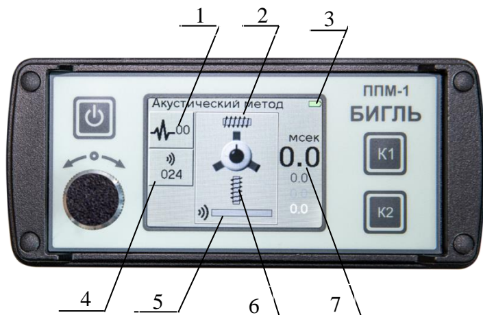
Рис.15 Основной экран приёмника ППМ-1 «Бигль» в акустическом режиме
